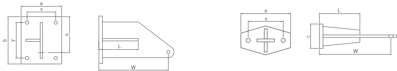
Kragarmkonsole
